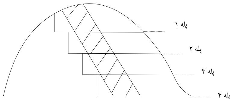
شکل ۳-۶- استخراج ذخایر برجسته به روش روباز پلکانی بخشی
