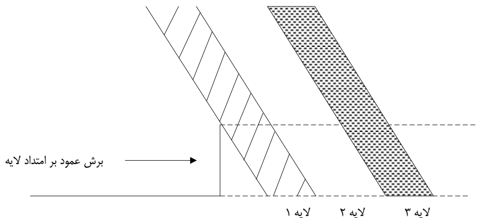
شکل ۴-۲- احداث برش اولیه در لایه‌های مرمريت شیب‌دار
