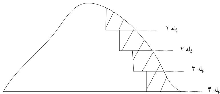
شکل ۳-۵- استخراج ذخایر برجسته به روش روباز پلکانی
