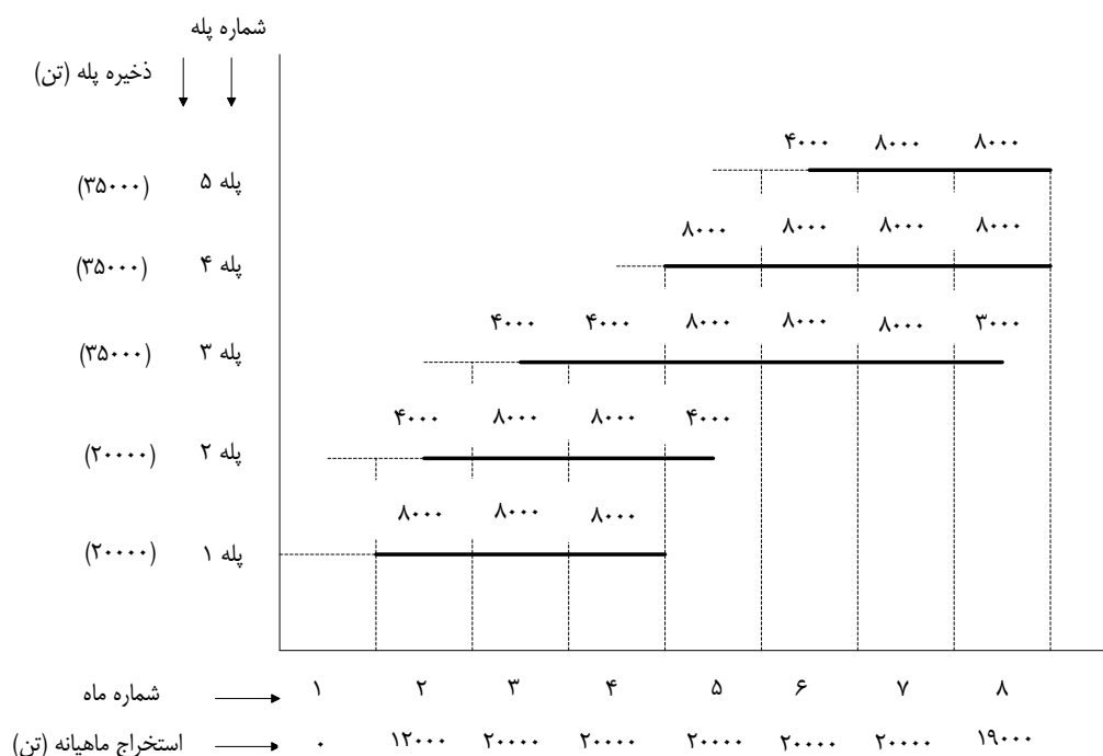
شکل ۶-۴- نمودار مراحل کار در یک معدن فرضی
