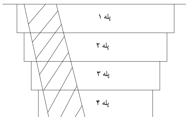
شکل ۳-۱۰- استخراج ذخایر پرشیب به روش پلکانی کلاسیک
